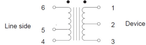
TEW4921-2
