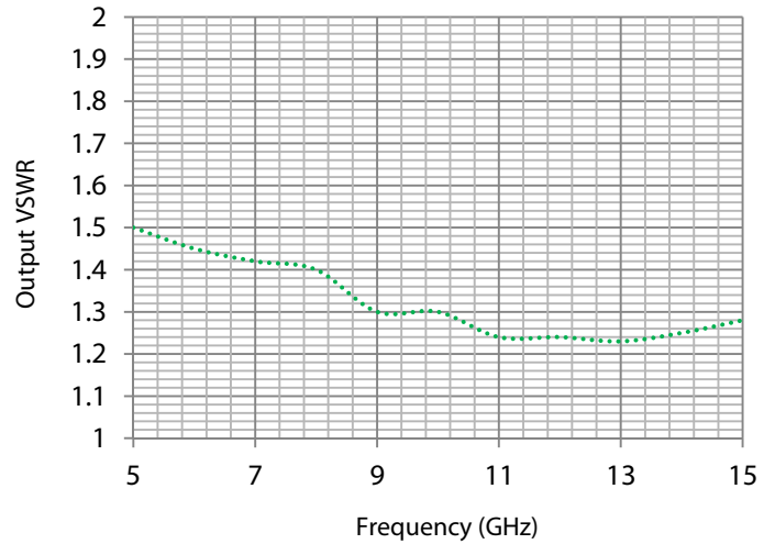
Output VSWR
