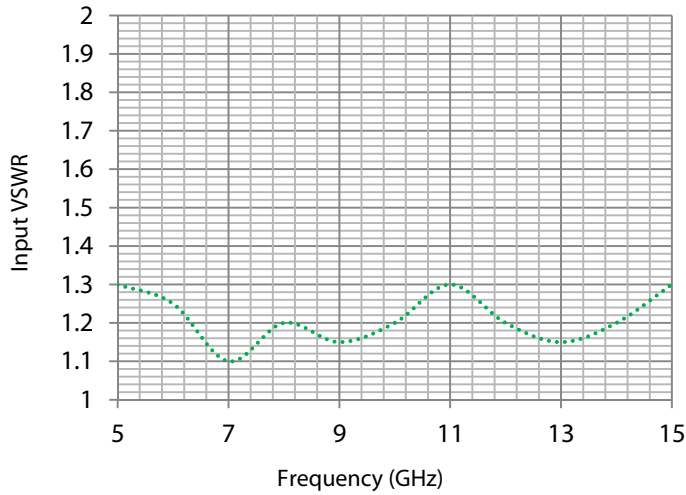
Input VSWR
