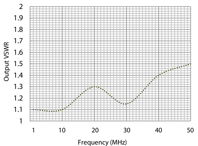
Output VSWR
