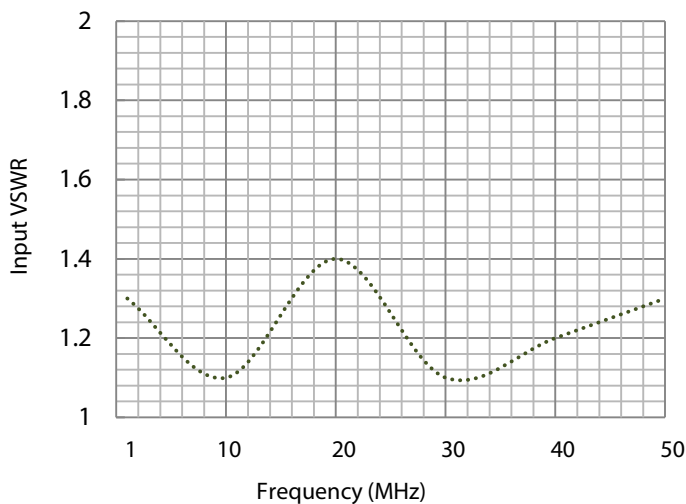
Input VSWR
