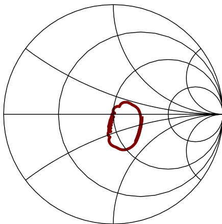
S11 (237.5-242.5 MHz)
